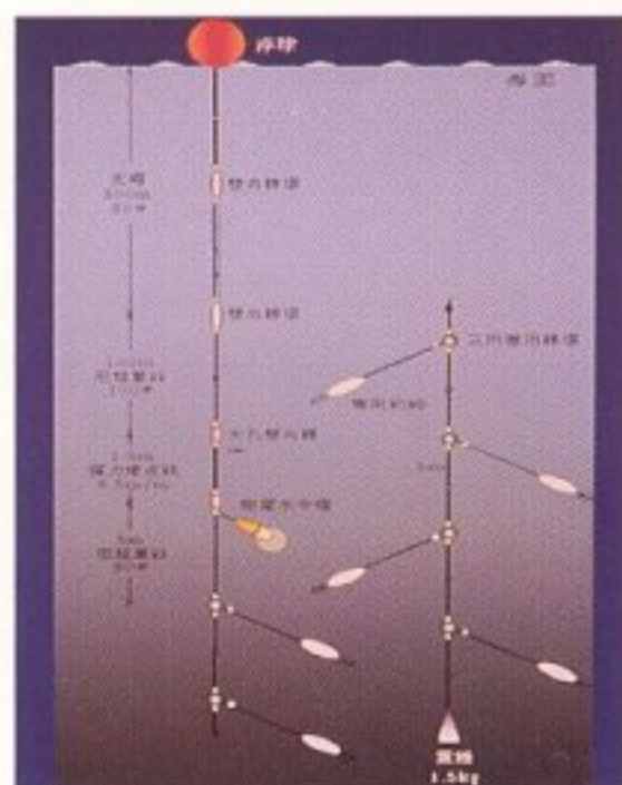
圖 2 菱鰭魷專用釣具構成圖
