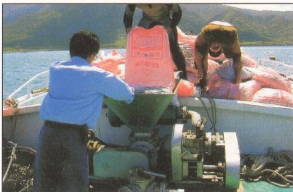
架設於船上之噴槍式自動投餌系統
