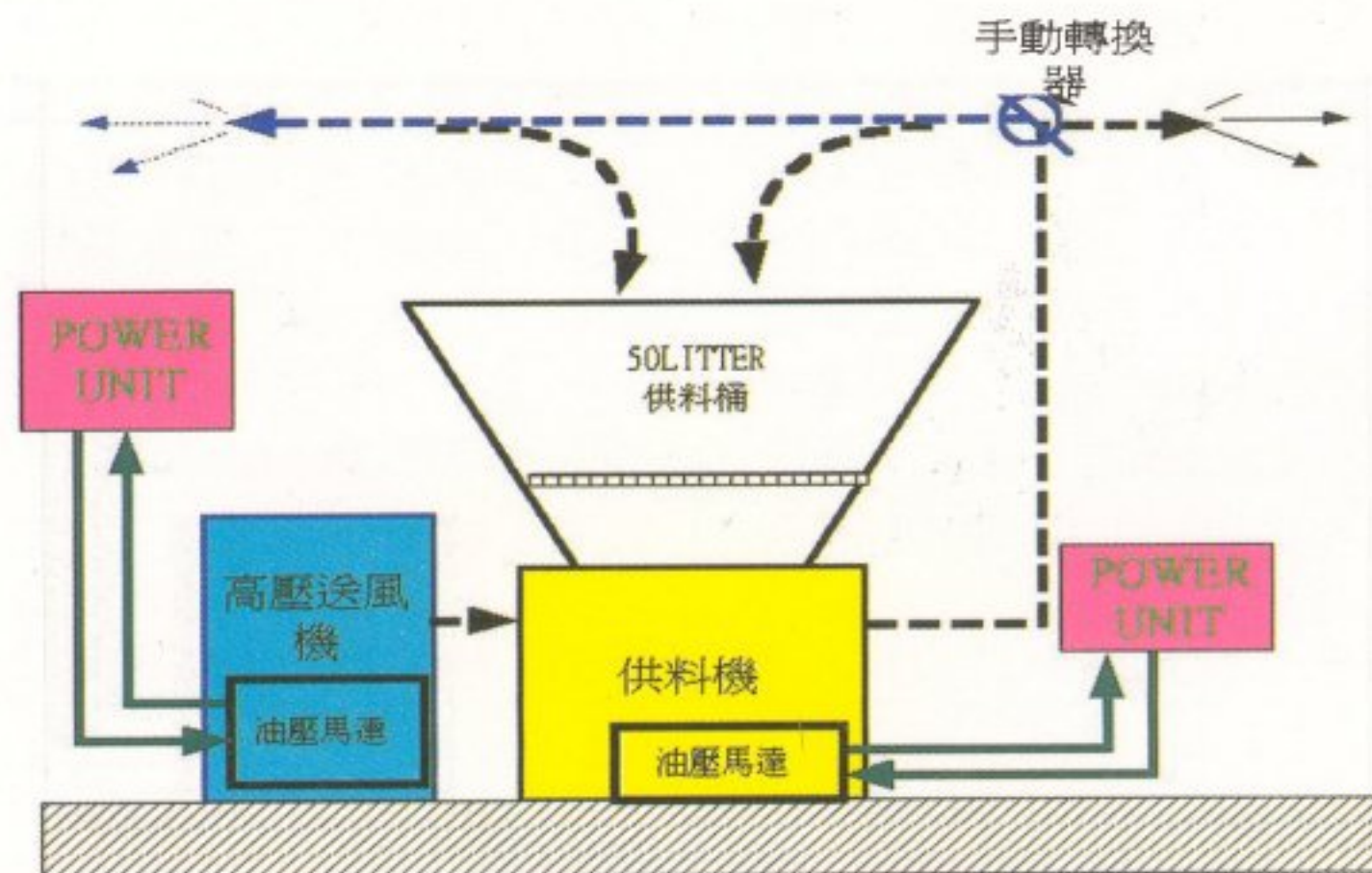
噴槍式海上箱網養殖自動投餌之系統架構
