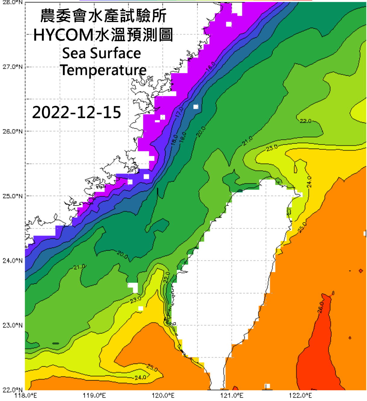
HYCOM-水溫模式預測圖 2022-12-14製圖
