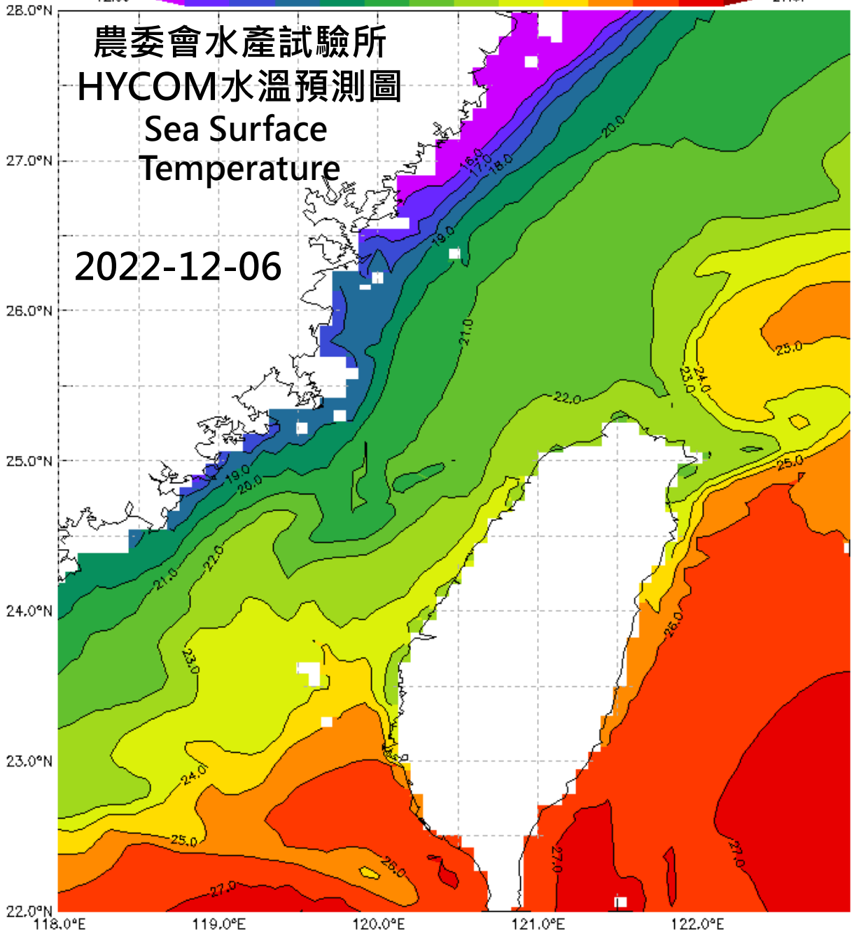
HYCOM-水溫模式預測圖 2022-12-06製圖
