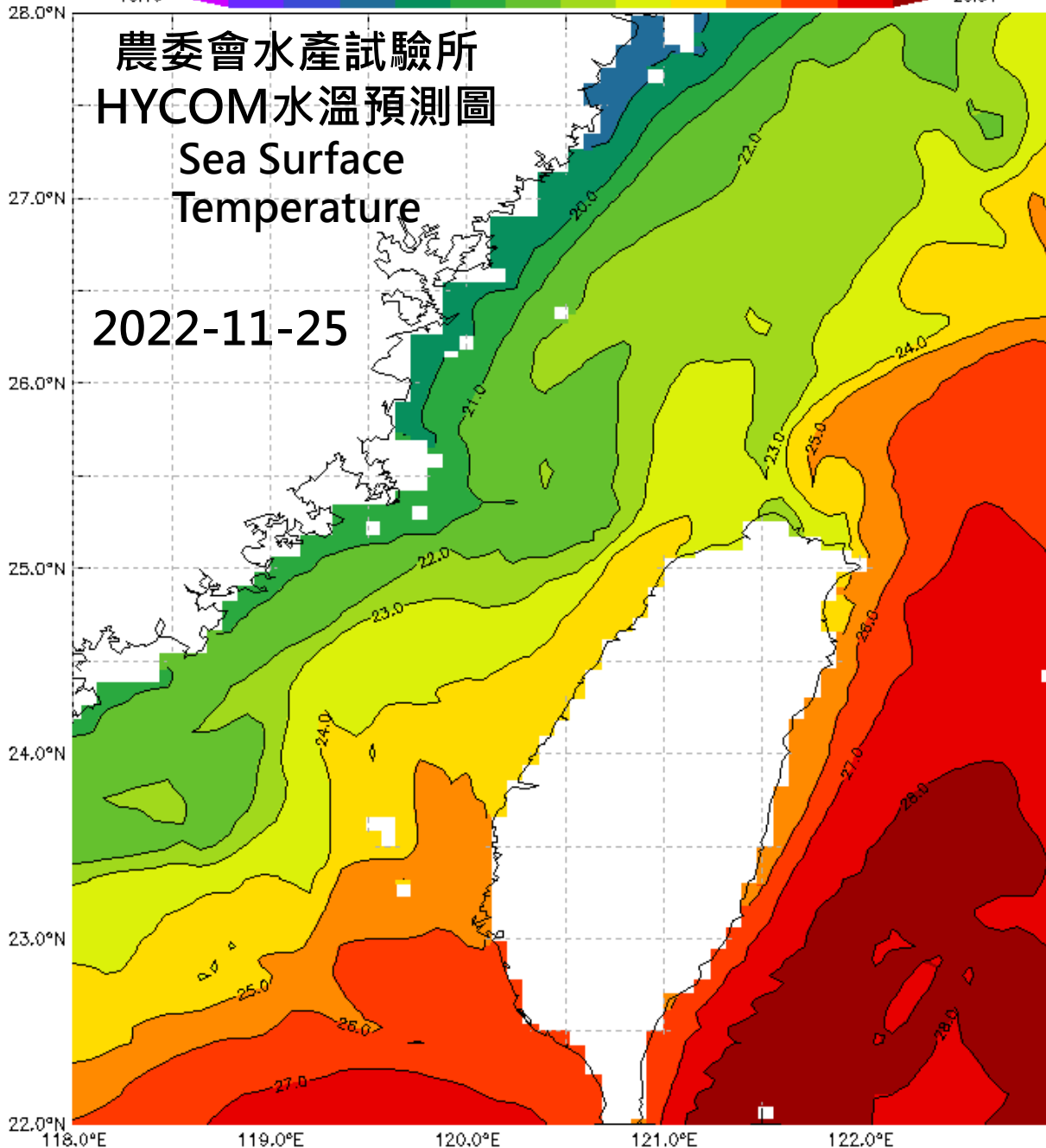
HYCOM-水溫模式預測圖 2022-11-25製圖
