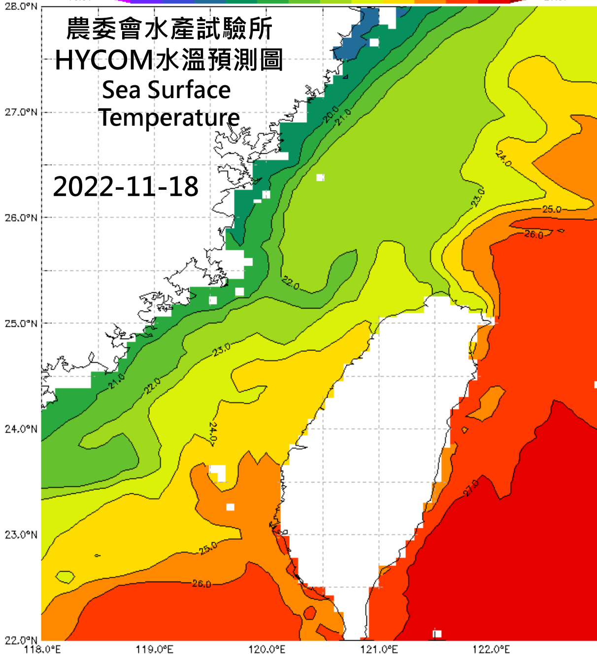
HYCOM-水溫模式預測圖 2022-11-18製圖
