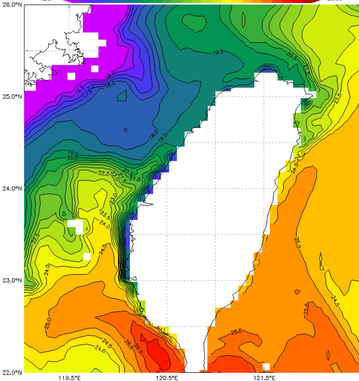
HYCOM-水溫模式預測圖 2022-12-19製圖
