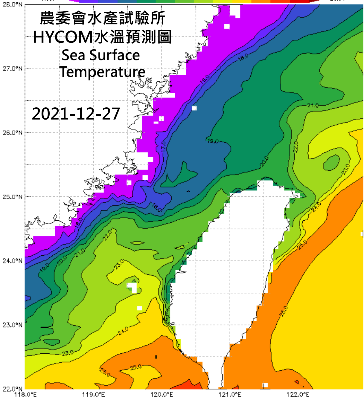
HYCOM-水溫模式預測圖 2021-12-24製作發布
