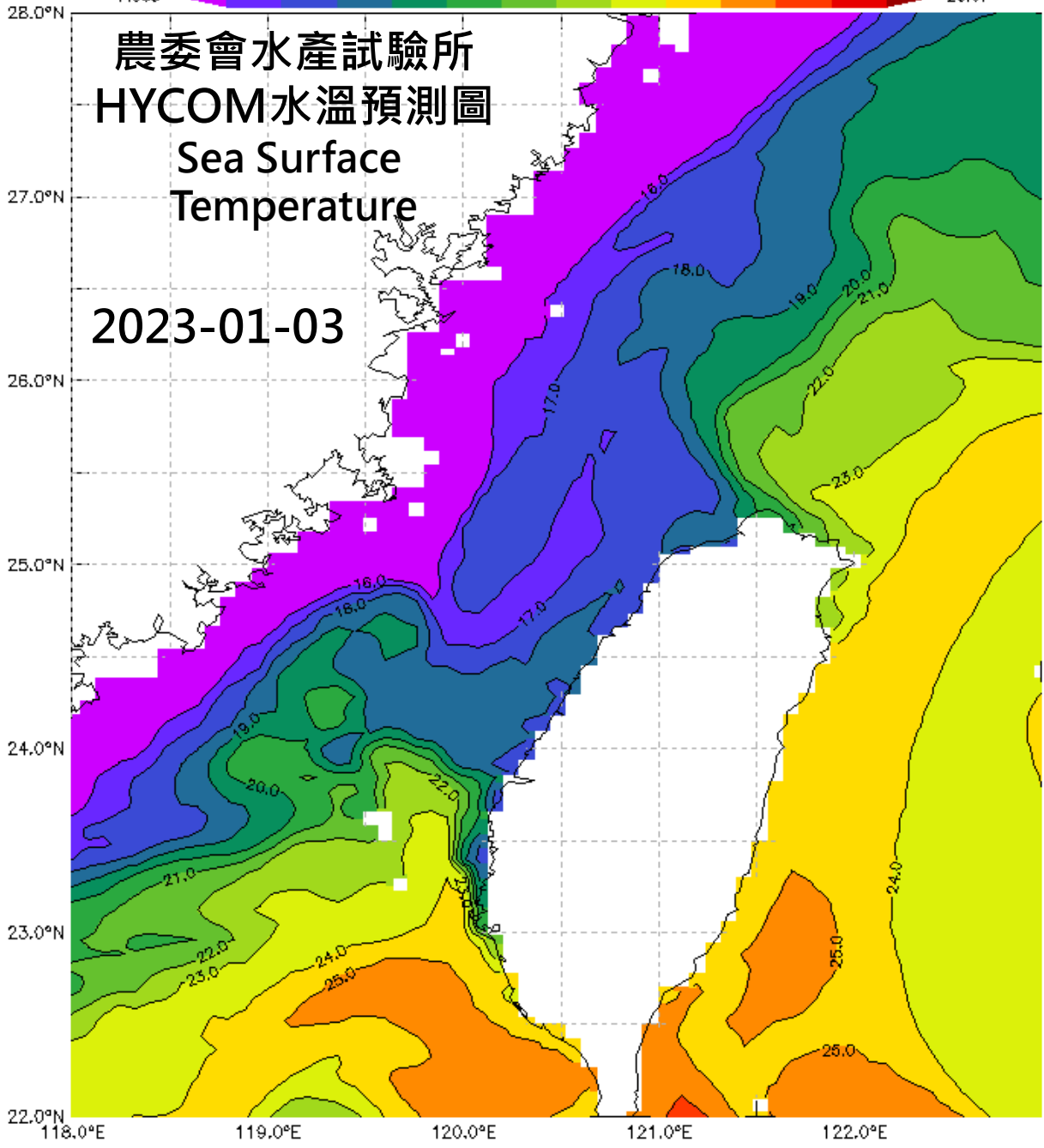
HYCOM-水溫模式預測圖 2023-01-03製圖
